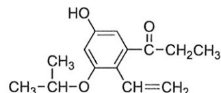
図1 構造式の例
