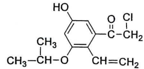
図1 構造式の例
